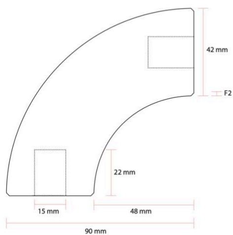
Zijaanzicht
