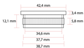
Zijaanzicht
