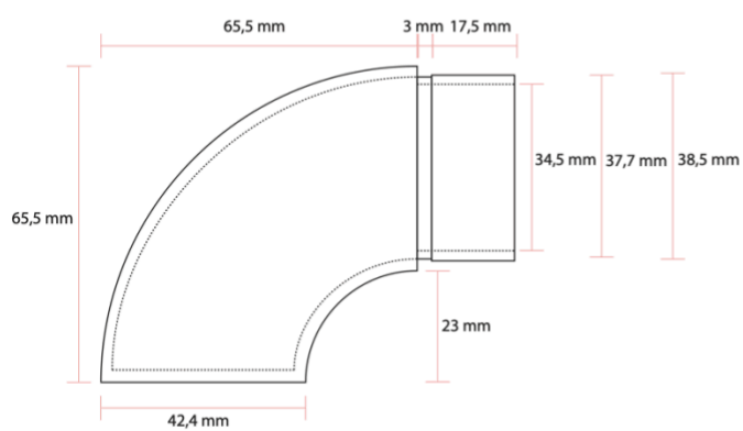
Zijaanzicht
